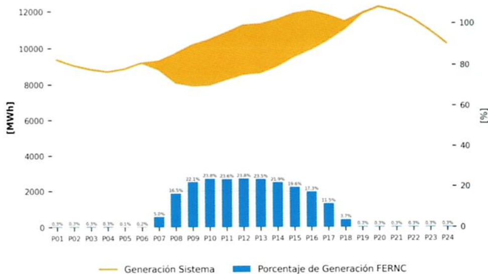
Figura 3. Curva de producción de energía eléctrica con fuentes solares fotovoltaicas instaladas en el Sistema Interconectado Nacional para el 11 de junio de 2026 (Elaboración propia a partir de información en SINERGOX)
